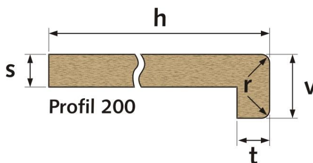
Osazení parapetu
