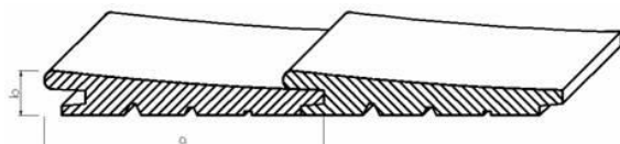
KLASICKÝ PROFIL
